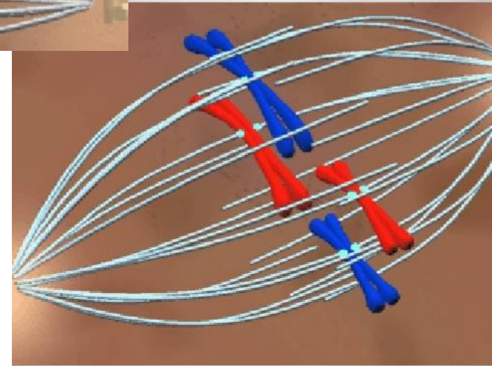
métaphase
