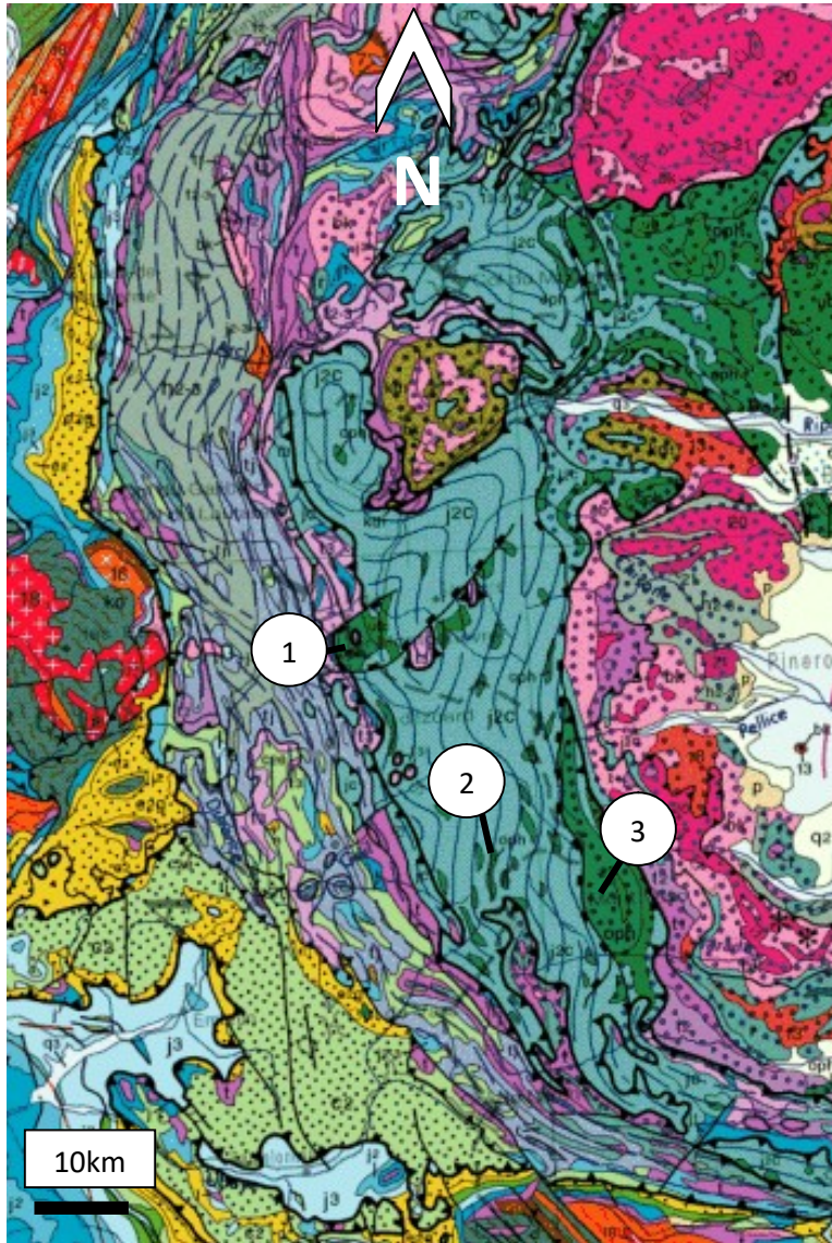
Extrait de la carte géologique de la France au millionième (BRGM, Esri)
