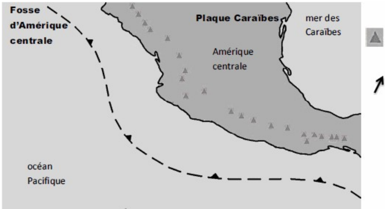
Contexte géologique de l'Amérique centrale
